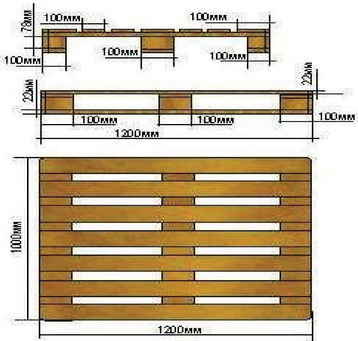
Рисунок 1 – чертеж поддона с указанием габаритных размеров
